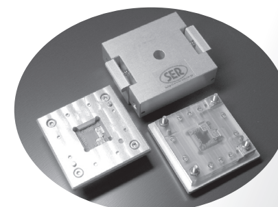
Zo=50Ω完全同軸ICソケット
