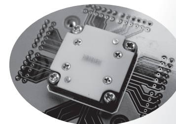
0.32mmボールピッチ WLCSPケルビンコネクタ
