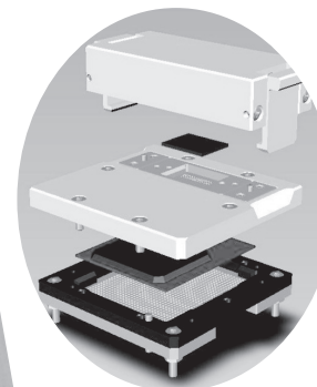
PoP LSI用 二重階層ICソケット
